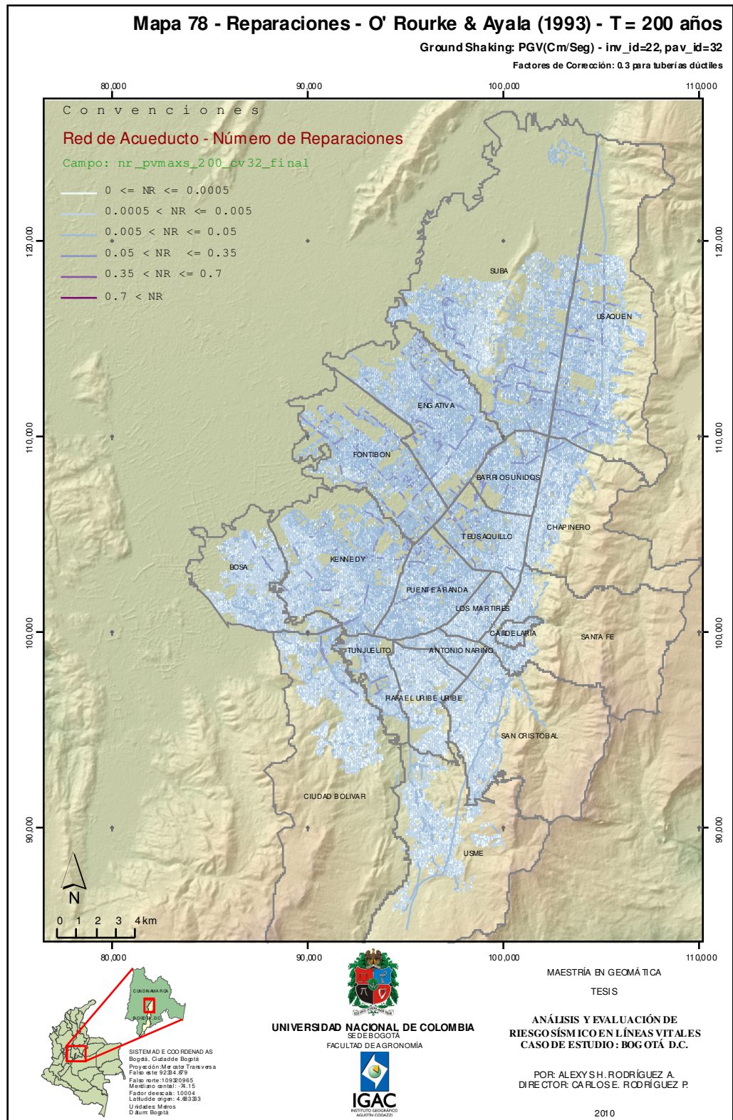
Figura 77. Mapa 78. Reparaciones red de acueducto. T= 200 años. (O'Rourke y Ayala, 1993)
