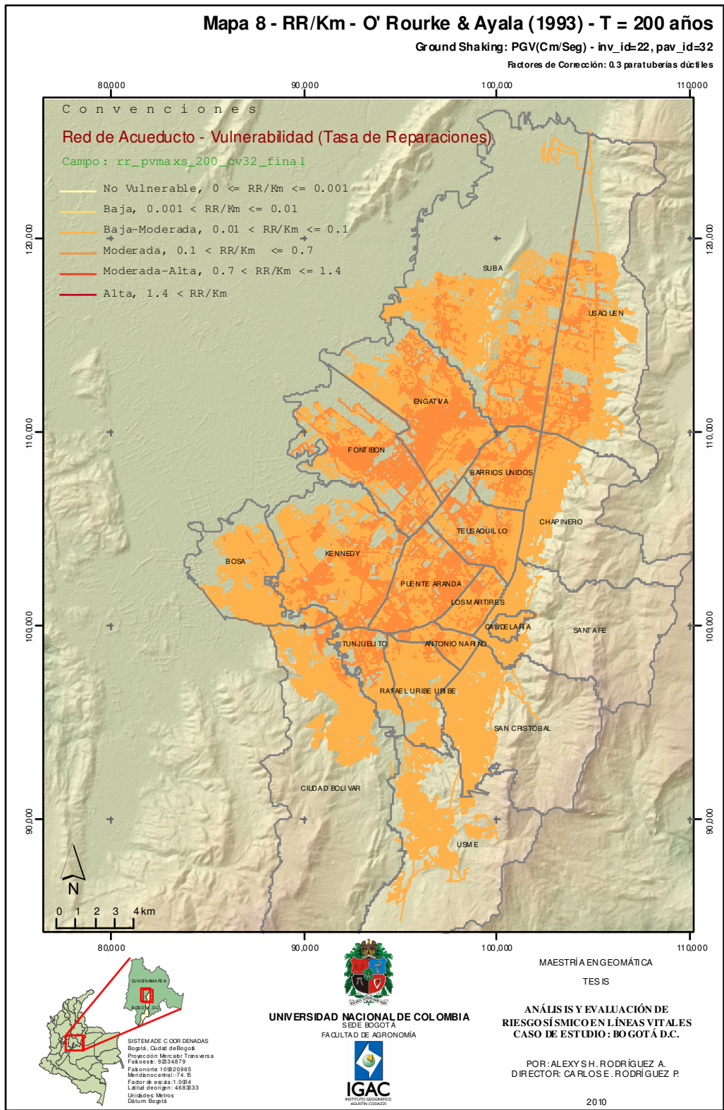
Figura 76. Mapa 8. Vulnerabilidad red de acueducto. T= 200 años. (O'Rourke y Ayala, 1993)
