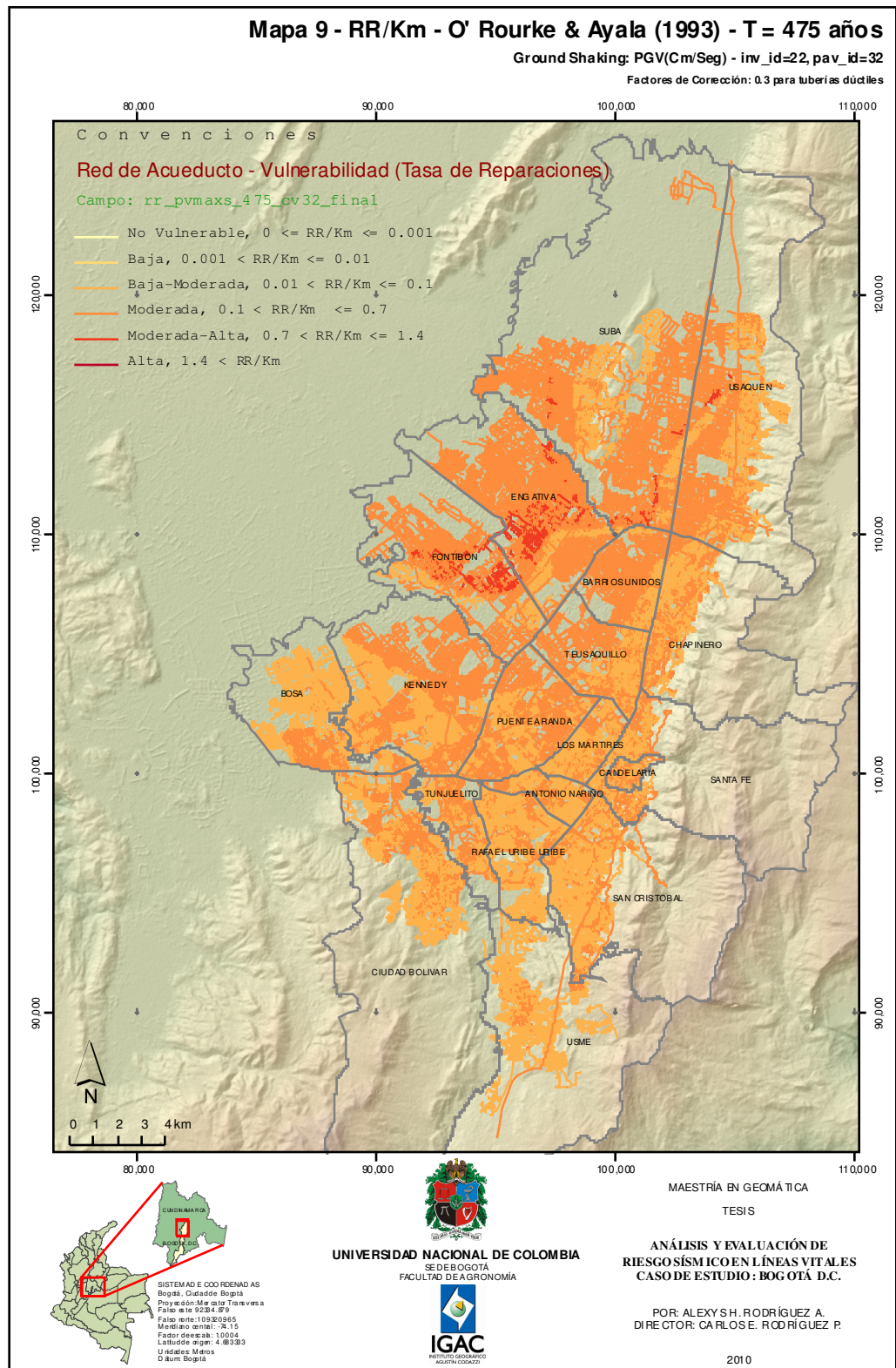
Figura 78. Mapa 9. Vulnerabilidad red de acueducto. T = 475 años. (O'Rourke y Ayala, 1993)
