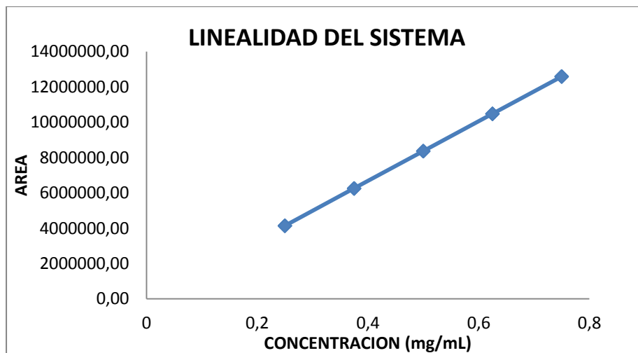
Figura 4-10. Curva de calibración de la linealidad del sistema
