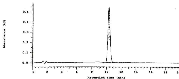
Figura 4-1. Cromatograma correspondiente a la hidrólisis ácida con HCl 1N.
