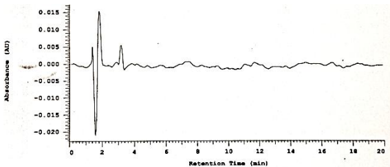
Figura 4-7. Cromatograma de Dextrosa al 5%.
