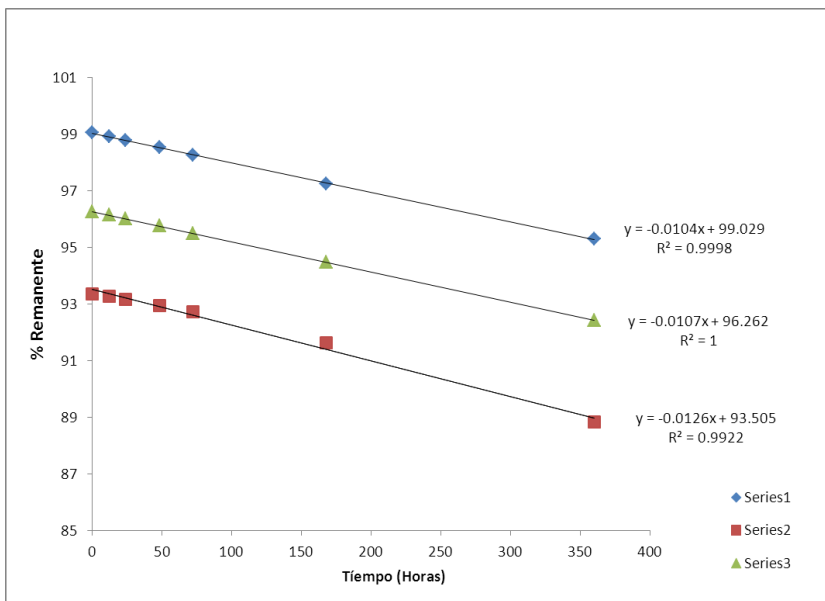
Figura 4-16. Gráfico de Regresión para Dextrosa al 5% a 30°C +/- 2°C
