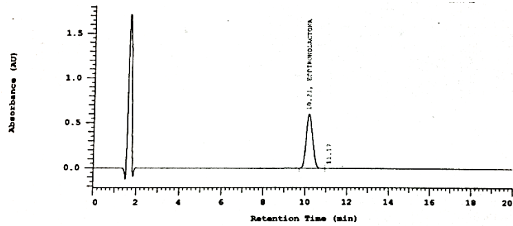
Figura 4-3. Cromatograma correspondiente a la degradación oxidativa.
