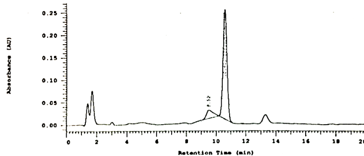
Figura 4-2. Cromatograma correspondiente a la hidrólisis básica con NaOH 1N.
