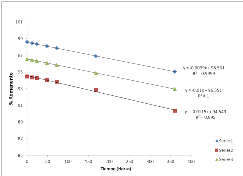
Figura 4-15. Gráfico de Regresión para Dextrosa al 5% a 5°C
