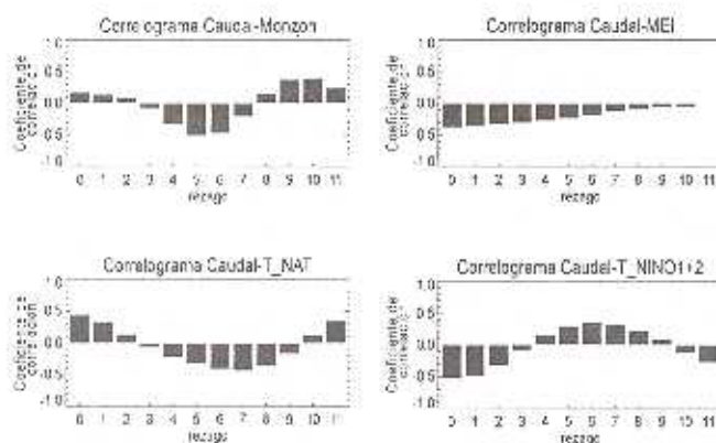
FIGURA 2. Correlogramas cruzados entre la serie del río Nare y las variables macroclimáticas.
