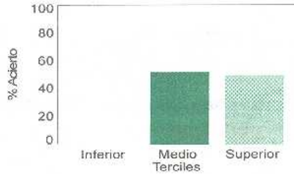
FIGURA 8. de aciertos agrupada por terciles suponiendo la climatología como predicción.
