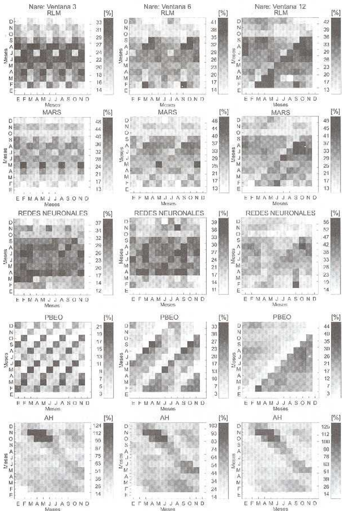
FIGURA 6. Porcentaje de RMS de las predicciones para el periodo de validación. Se tiene en las absisas se tiene el mes de inicio de la predicción y en las ordenadas el mes predicho. De izquierda a derecha se tienen los errores para diferentes ventanas de predicción 3, 6 y 12, respectivamente. De arriba hacia abajo se tienen los resultados al emplear los diferentes modelos RLM, MARS, Redes , Neuronales, PREBEO y AH
